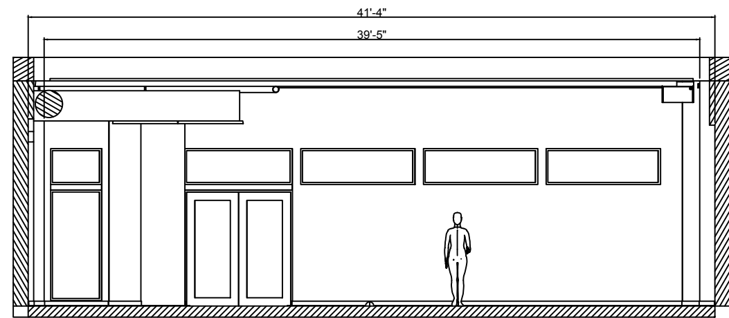
COUPE A-A
