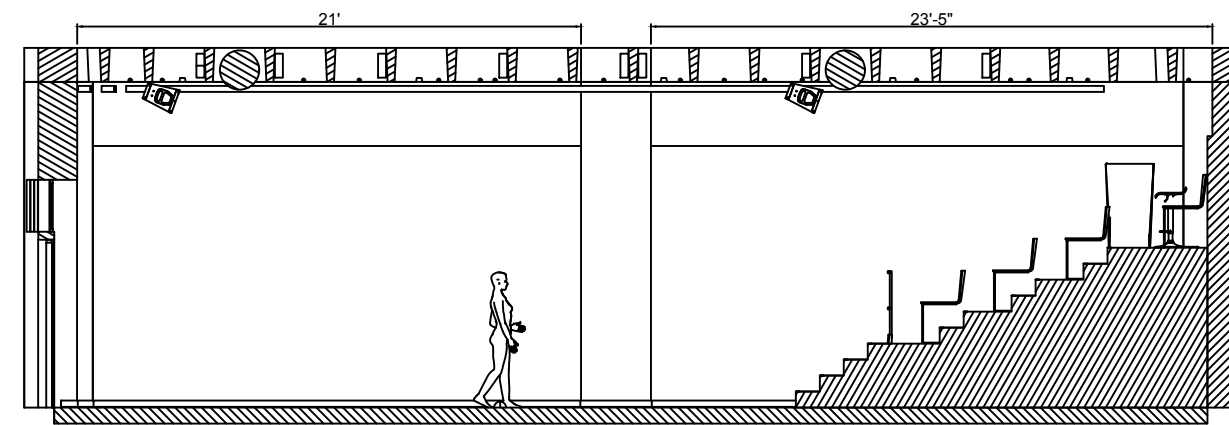
COUPE C-C
