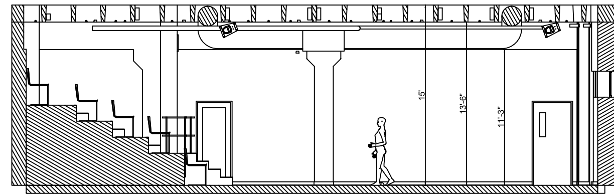
COUPE D-D
