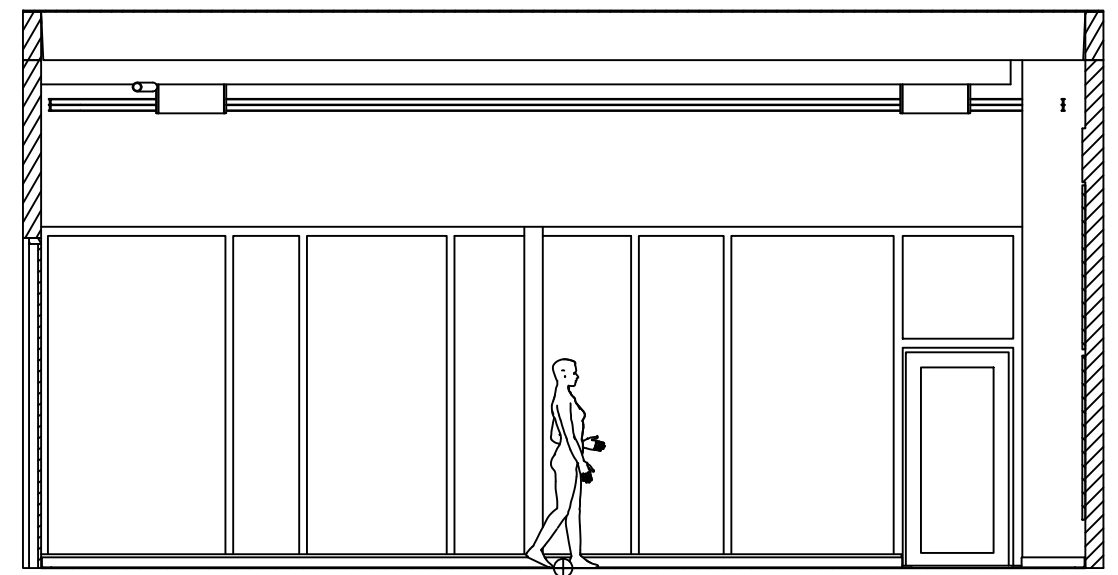
COUPE D-D
