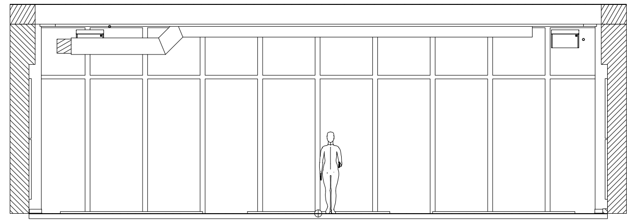
COUPE D-D
