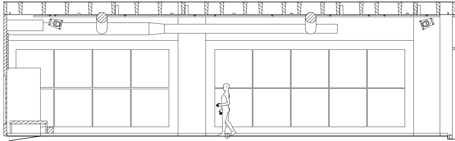
COUPE A-A
